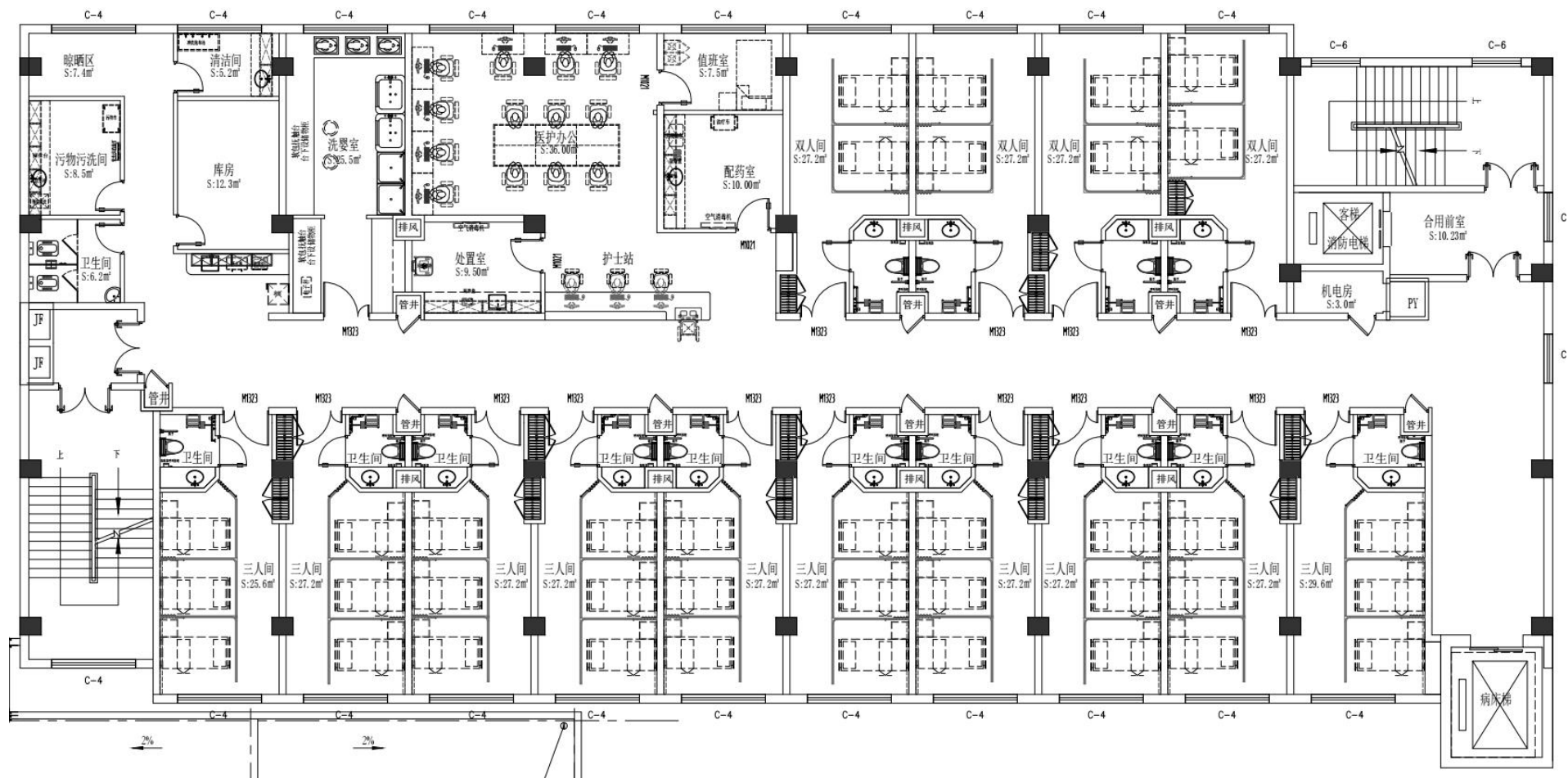
附图 3-4 3~5F 平面布置图
