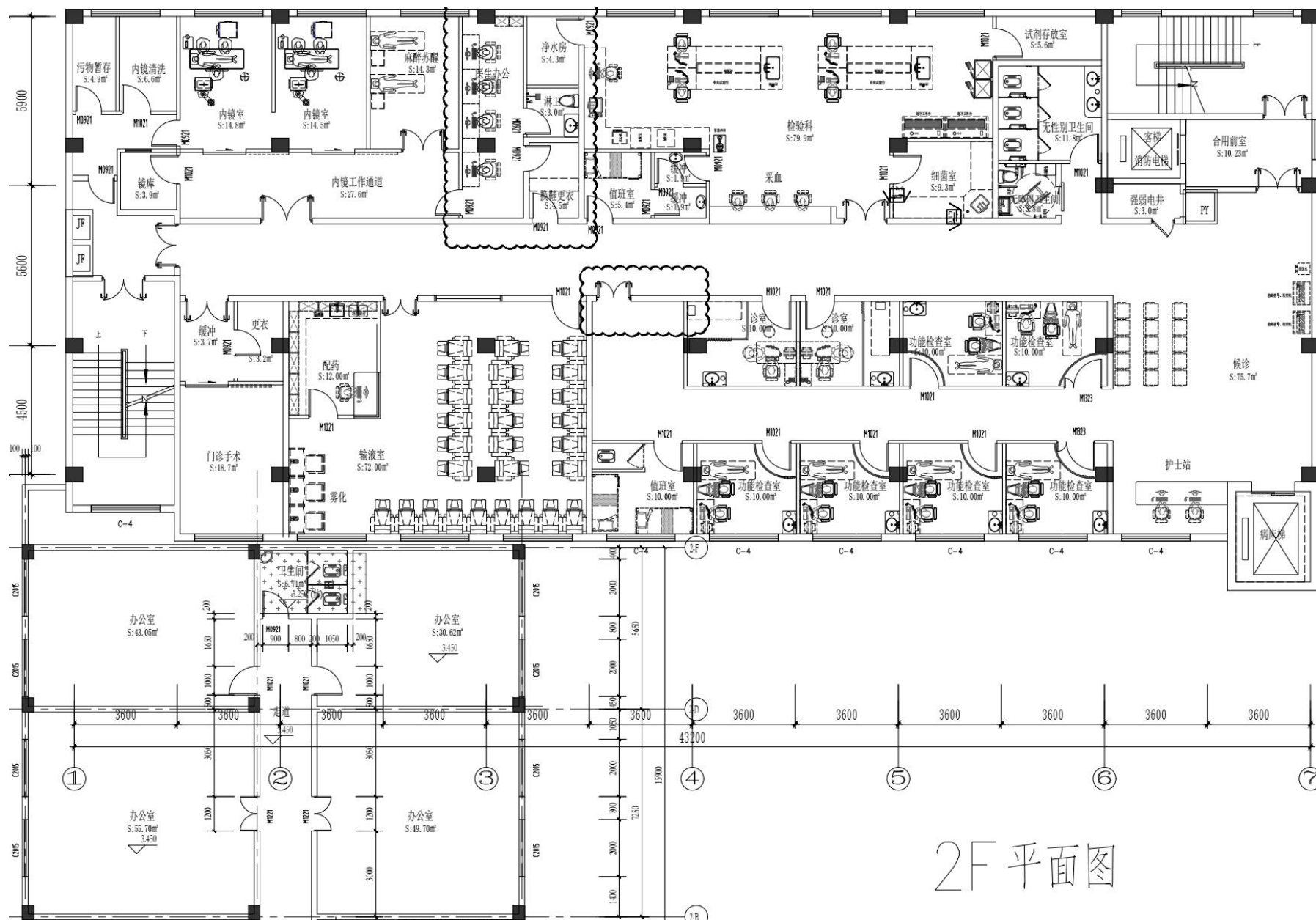
附图 3-3 2F 平面布置图
