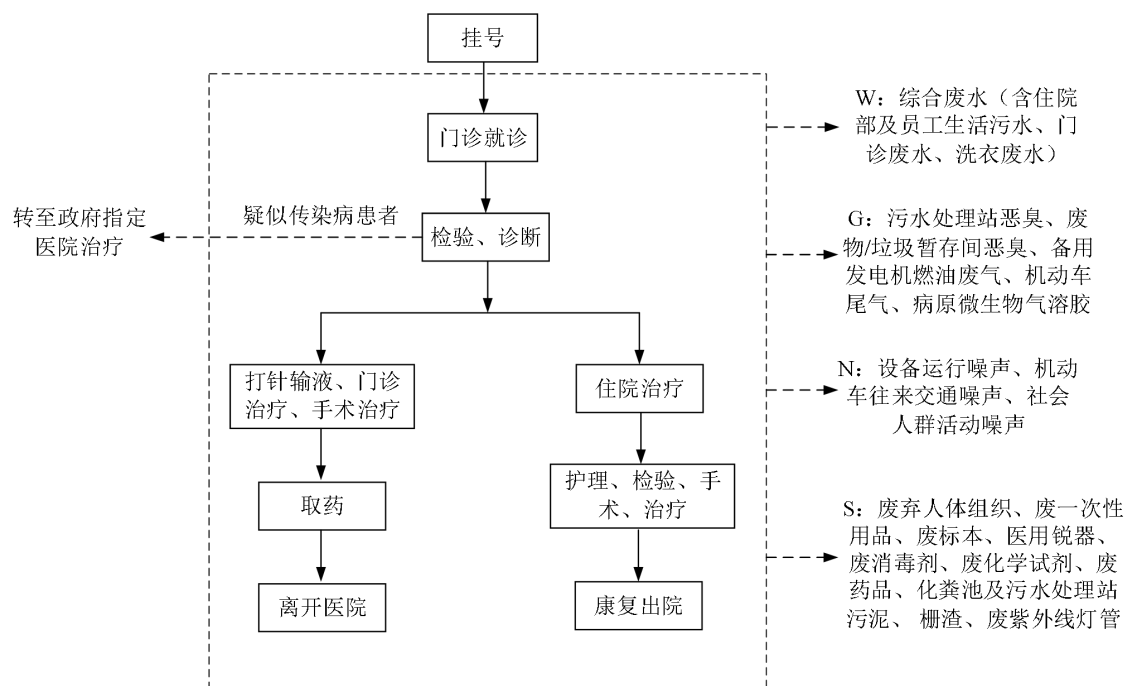
图2-3 运营期工艺流程及产污节点图
