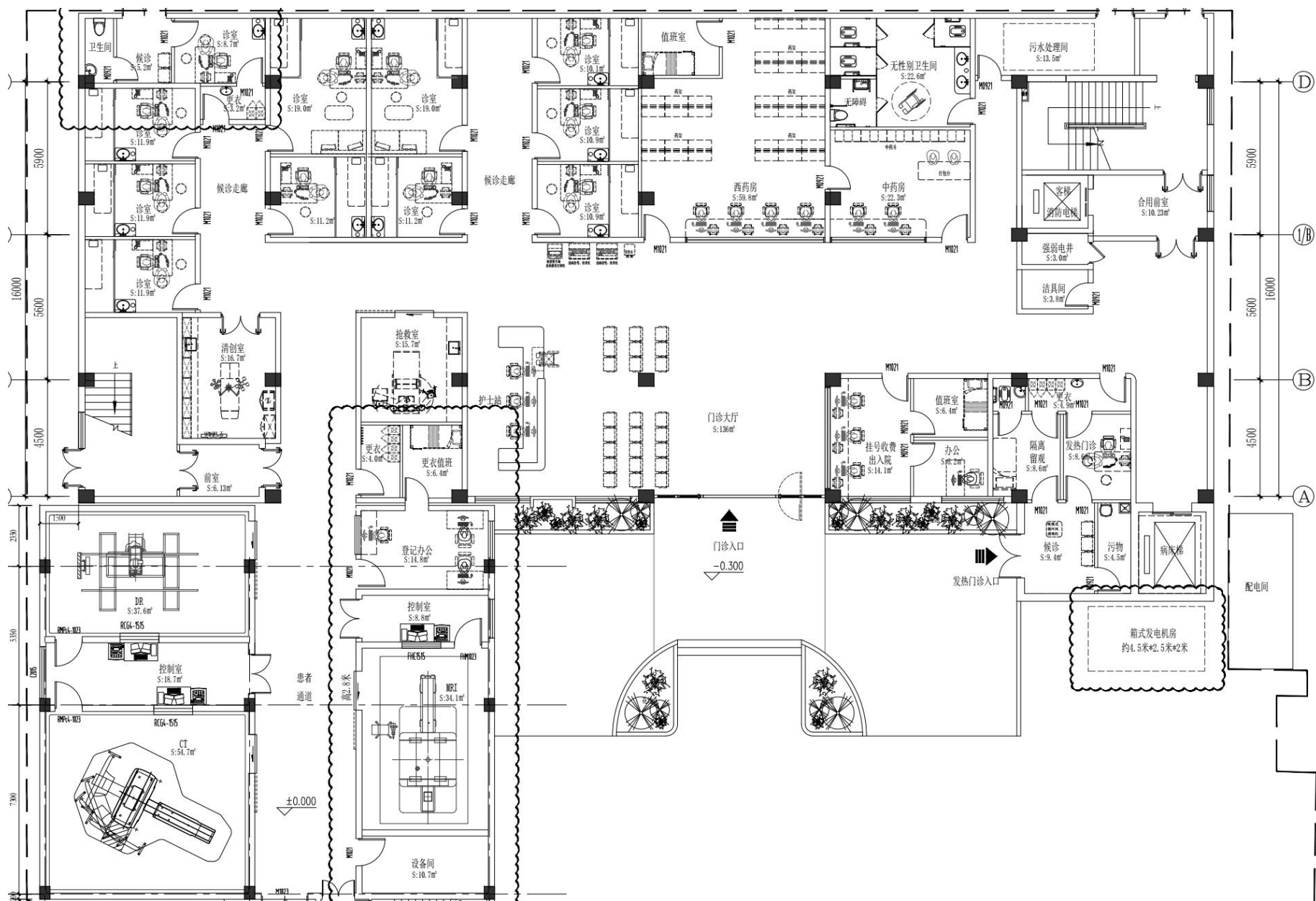
附图 3-2 1F 平面布置图
