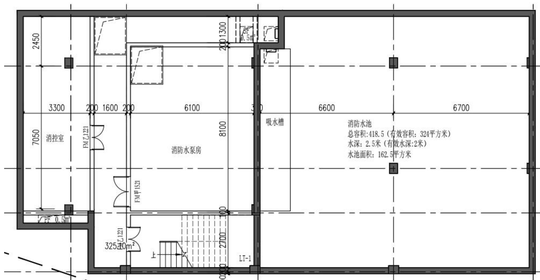
附图 3-1 地下室平面布置图
